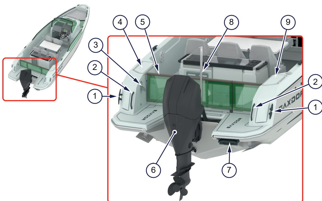
Kuva 4.6 - Uimatasanteen komponentit
