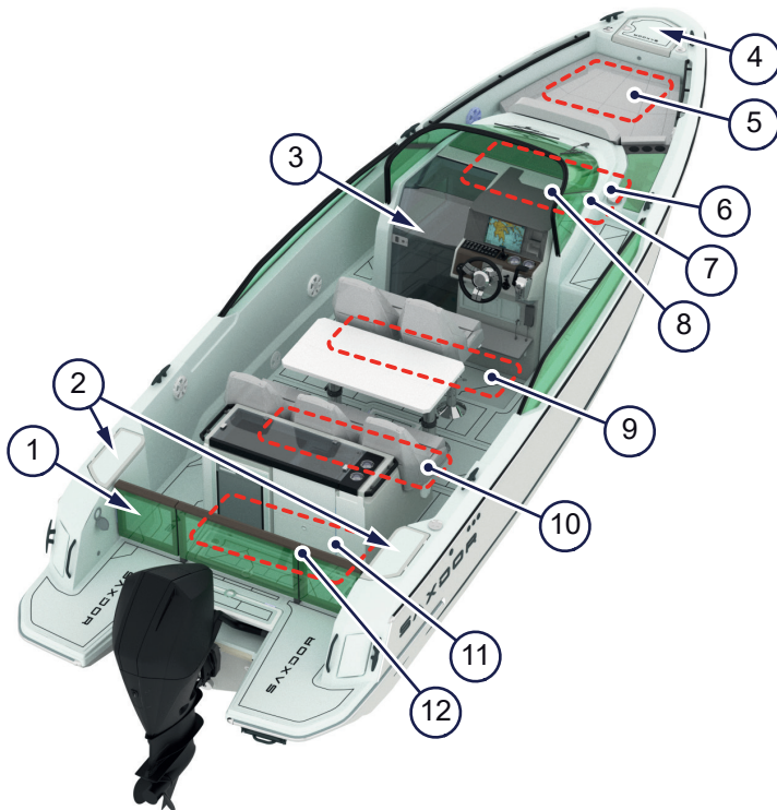
Kuva 4.22 - Luukut
