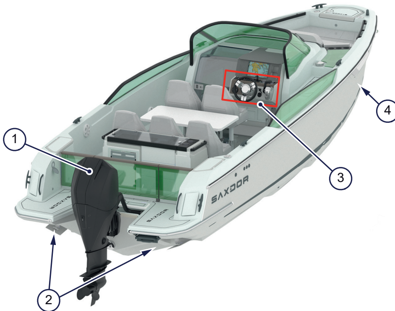
Kuva 5.2 - Moottori ja ohjaus
