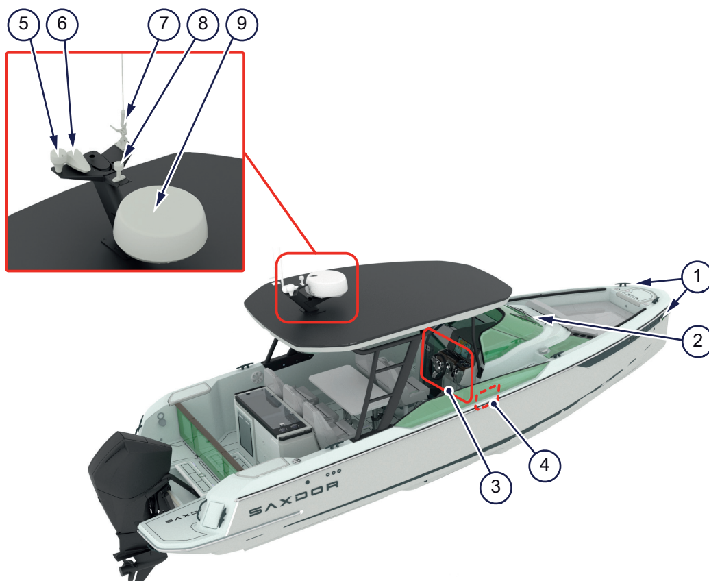
Kuva 5.7 - Navigointivarusteet
