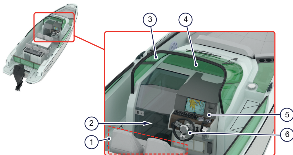
Kuva 4.4 - Ohjaamo
