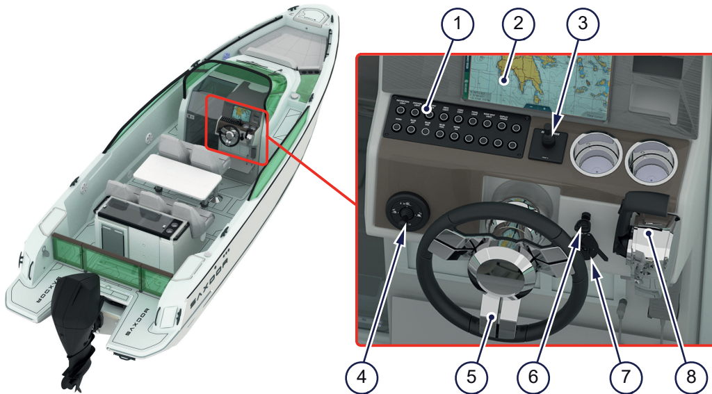
Kuva 4.8 - Ohjauspisteen hallintalaitteet
