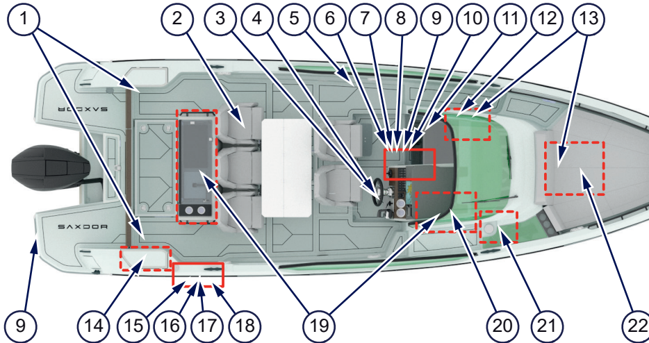
Kuva 4.18 - Veneen turvamerkintöjen sijainti
