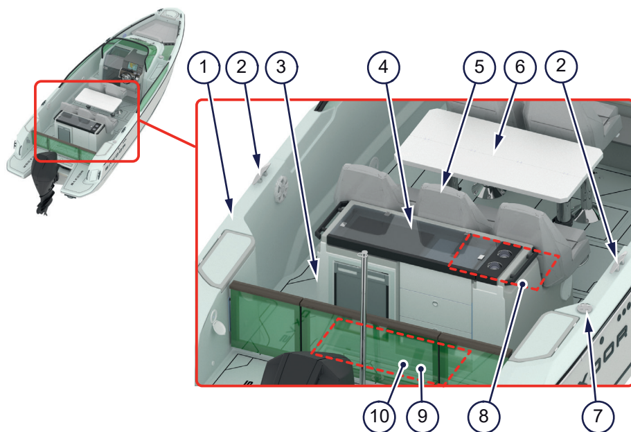
Kuva 4.5 - Peräkansi
