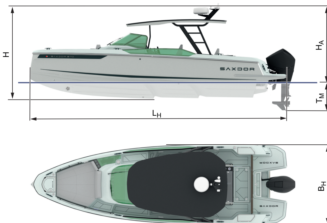
Kuva 8.1 - Saxdor 270 GTO/R:n mitat
